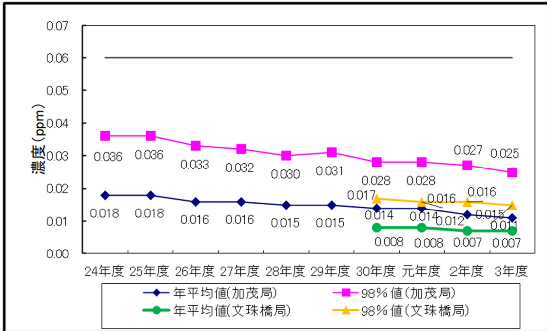
【図 5-12 加茂自動車排気ガス測定局と川西文珠橋自動車排気ガス測定局の二酸化窒素濃度経年変化（年平均値及び日平均値の年間 98%値）】
